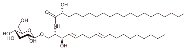
フィトセラマイドに含まれる主要グルコシルセラミドの構造式
